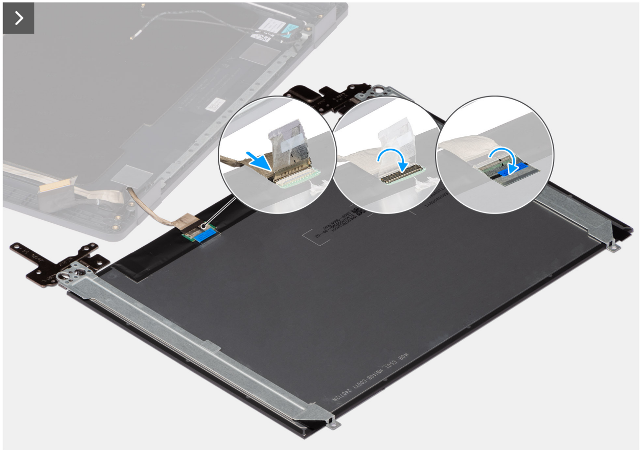
Abbildung 79. Installieren der Bildschirmbaugruppe
