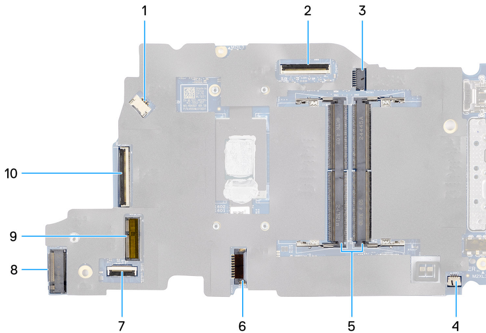
Abbildung 42. Hauptplattenanschlüsse
