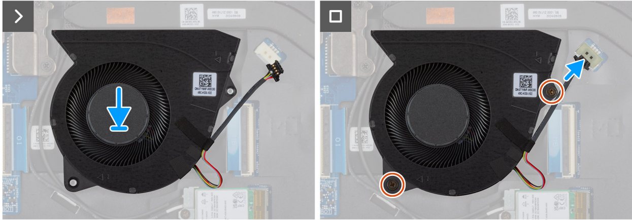
Abbildung 31. Einbauen des Lüfters
