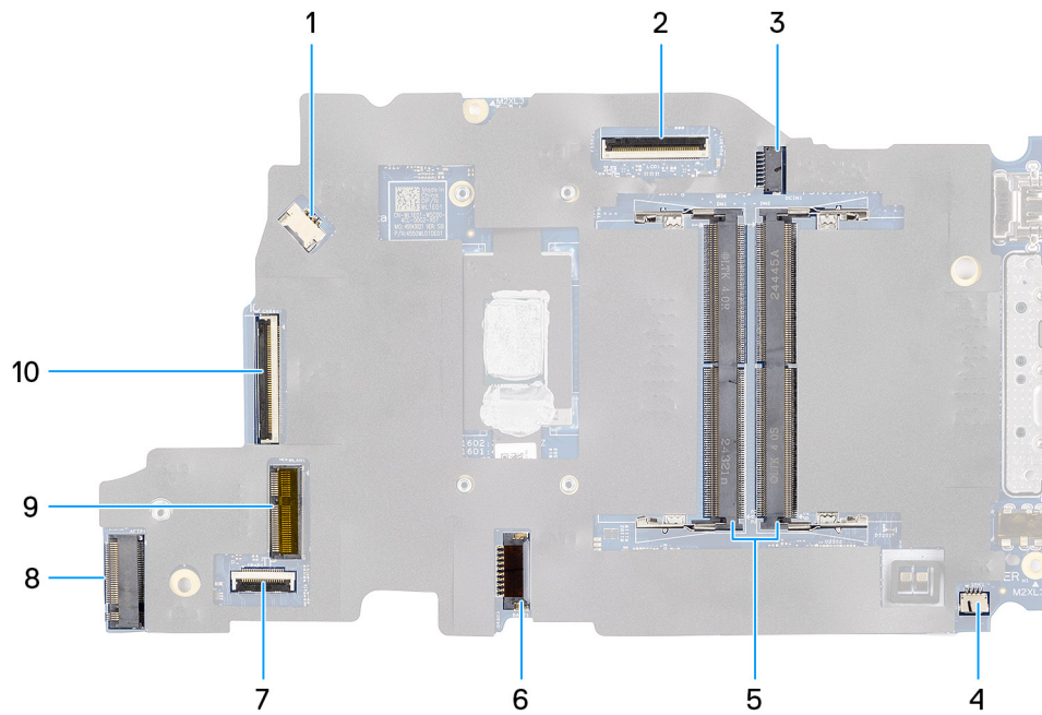
Abbildung 45. Hauptplattenanschlüsse
