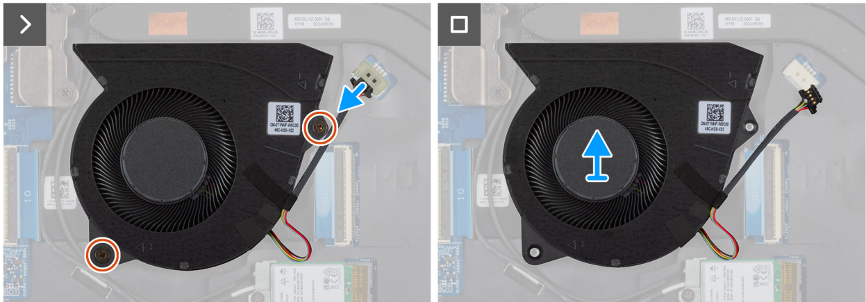
Abbildung 30. Entfernen des Lüfters
